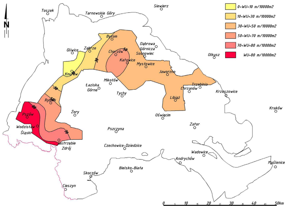
Rys. 3. Mapa zmian wartości wskaźnika zuskokowania W_U w GZW
